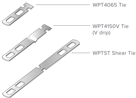
WPT4065 Tie
